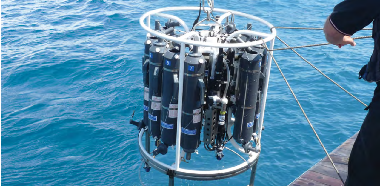
דגימת מי הים הפתוח במפרץ חיפה, מאי 2012. צבעם הכחול של המים מלמד על מיעוט חומרי הזנה במים ועל ריכוזי מיקרו־אצות נמוכים. מתקן הדגימה (ידוזה) כולל בקבוקים לדגימת מי הים ומכשור למדידת לחץ (עומק), טמפרטורה, מליחות וריכוזי כלורופיל | צילום: נגה סטמבלר
