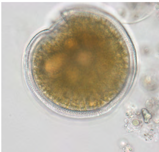
Gambierdiscus cf. excentricus - דינופלגלט שוכן קרקעית ממפרץ אילת. רחבו 75 מיקרון | צילום: Jacob Larsen
