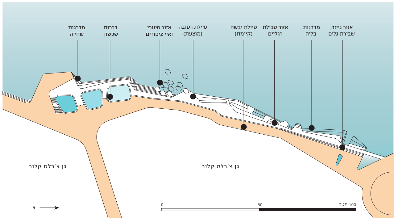
איור 1. תכנית הפיתוח של הגן הכחול מצפון לגן צ'רלס קלור, ומדרום לדולפינריום בתל-אביב-יפו. תכנון: יאשה גרובמן ורועי קוזלובסקי.
