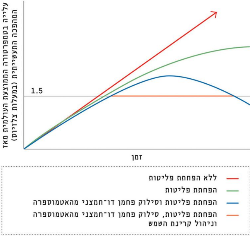
איור 1. מהלך סכמטי של הטמפרטורה העולמית כפונקציה של הזמן כתלות באופני התנהלות שונים לגבי הפחתת פליטת גזי חממה ושימוש באסטרטגיות של הנדסת אקלים
