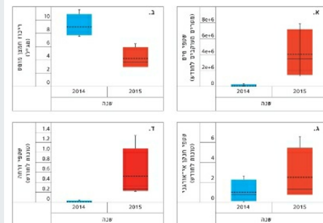
איור 5. נמונים מסכמים 2014 ו-2015: תקופה מורגבת הזרמות לעומת תקופה מעוטת הזרמות א. שטפי מים חודשיים שזרמו אל הור השפך; ב. ריכוזי חמצן וממוצע על כל השפך; ג. שטפים חודשיים של חנקן אי-אורגני; ד. זרחה בכניסה לשפך ליד ג'ית 4. בכל עמודה מוצגים הערך המרבי, המזרני (נקודת אכזיב), הממוצע (בקו מקוקו), החציון (בקו רציף) והרכיבים (החוסר השטח הצבעוני) עבור ינואר עד אפריל של שנת 2014 ומכללה לעומת 2015 (אדום). השטפים חוטבו כמפלח הריכוז שנמדד בראש האסטואר במהלך החודש בסכום הספיקות החודשי מסודרות רשות המים.
