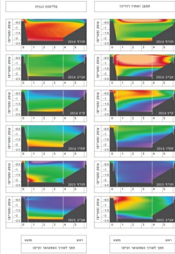
איור 3. ממוצעים חודשיים של נמוני חמצן ומליחות לאורך אקסטר אלכסנדר, ממוצא האקסטר לים (משמאל) ועד ראשו במעלה הנחל (מימין) נקודות הדגימה בפועל מיוצגות כנקודות לבנות. נערכה אינטרפולציה בין נקודות הדגימה בעזרת חוכנת Ocean Data View. ציר X – מרחק מהים; ציר Y – עומק. ערכי רוויית החמצן והמליחות מוצגים לפי מדרג הצבעים המוצג במקרא. חורף 2014 (ינואר-מרץ); אביב 2014 (אפריל-יוני); קיץ 2014 (יולי-ספטמבר); סתיו 2014 (אוקטובר-דצמבר); חורף 2015 (ינואר-מרץ); אביב 2015 (אפריל-יוני).
