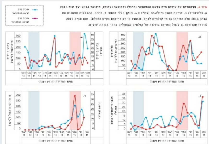
איור 4 פרמטרים של איכות מים בראש האסטואר (כחול) ובמוצא (אדום), מינואר 2014 ועד יוני 2015
