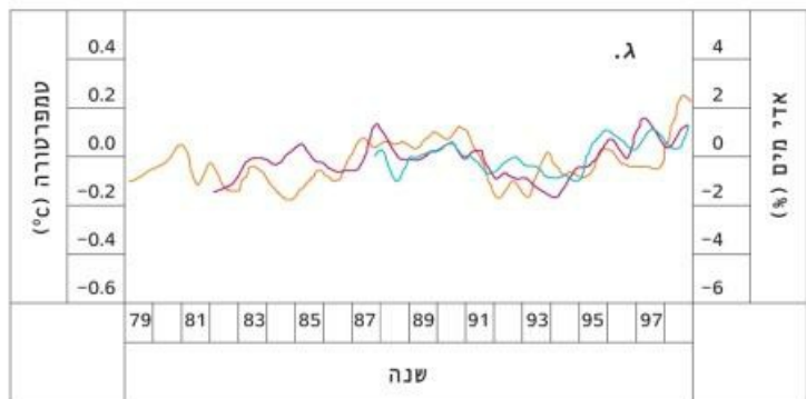
— T_A טמפרטורת האוויר — T_s טמפרטורת פני הים — W ריכוז אדי מים
