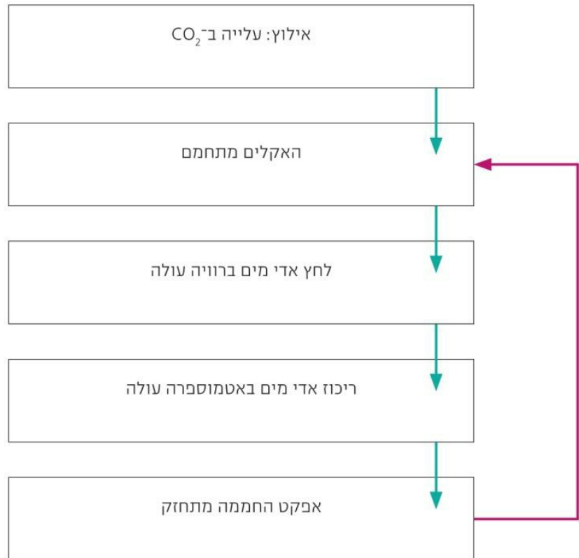
איור 1 משוב אדי מים
