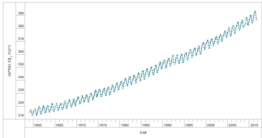
איור 3א. ריכוז חודשי ממוצע של פחמן דו-חמצני בפסגת המאונה לואה, הוואי לקוח מאתר מכון המחקר Scripps באוניברסיטת סן דייגו, קליפורניה [20].
