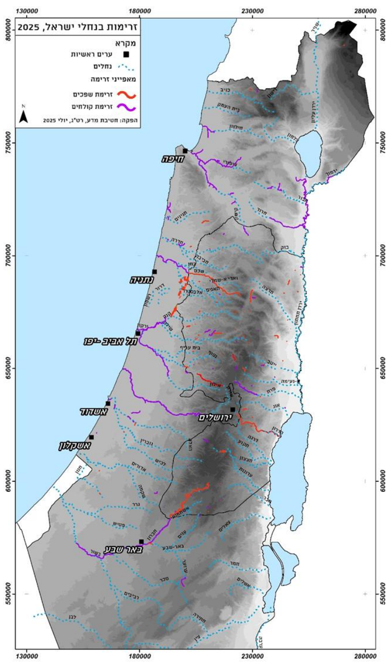
איור נ1. הזרמות קבועות של עודפי קולחים בנחלי ישראל, נכון לשנת 2025
